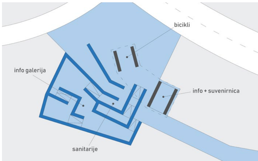
Slika 7. Kopneni ulaz — info punkt — tlocrt
