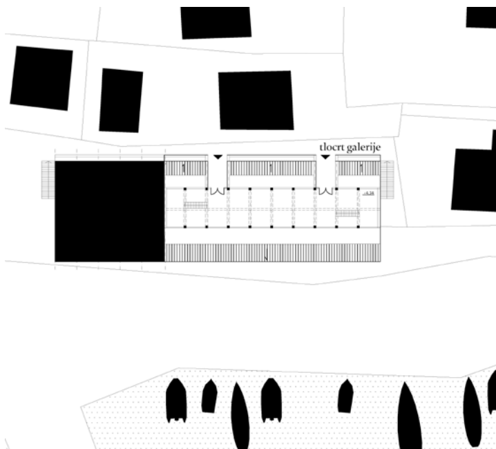
Slika 5. Tlocrt galerije
